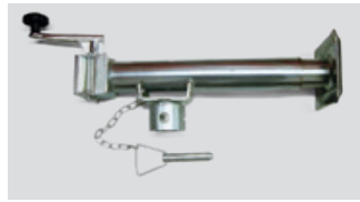
402616.001 Stützfuß klappbar LR3102 vz 1300kg 57x 430
